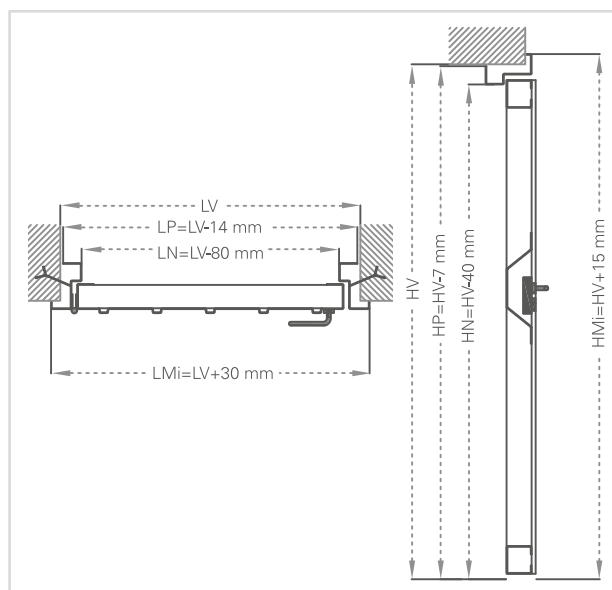
MOD. LIGHT - TIRARE
