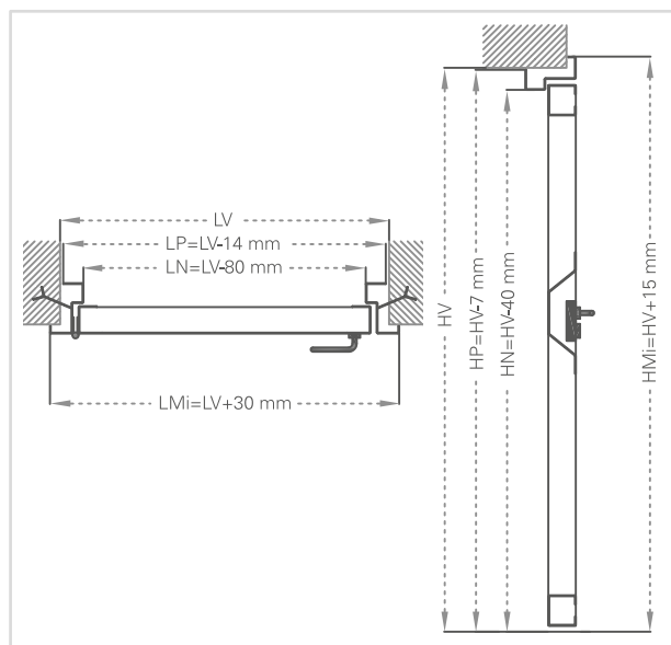
MOD. STRONG - TIRARE
