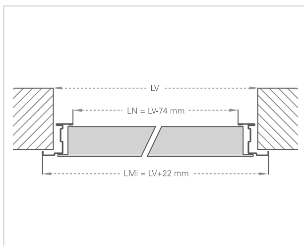
MOD. MULTIUSO - SEZIONE ORIZZONTALE
